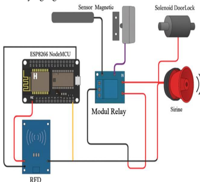
Gambar 2. Perancangan Rangkaian
